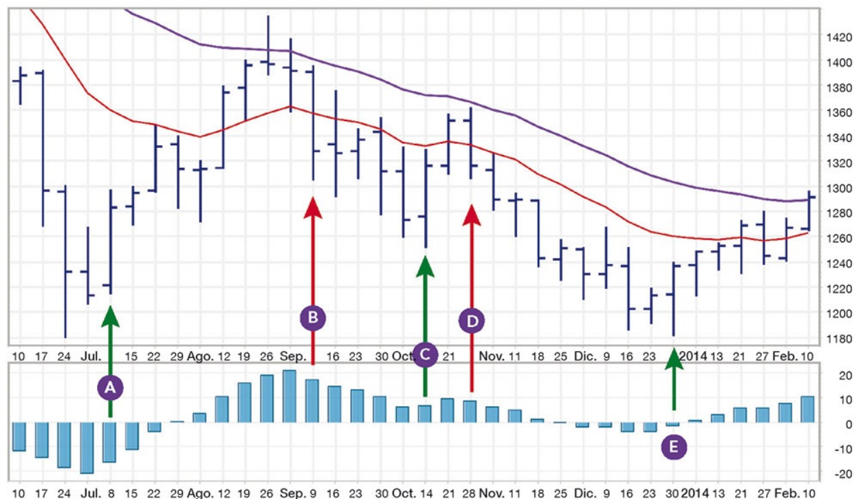
FIGURA 39.1 Oro semanal, con MME de 26 y 13 e histograma MACD (12-26-9) (Gráfico de StockCharts.com).
